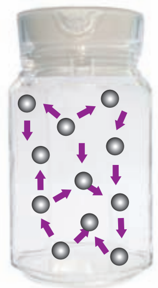
Aire encerrado en un frasco. Las pelotas representan las moléculas del aire y las flechas son vectores que representan la magnitud y la dirección de la velocidad de las moléculas.
